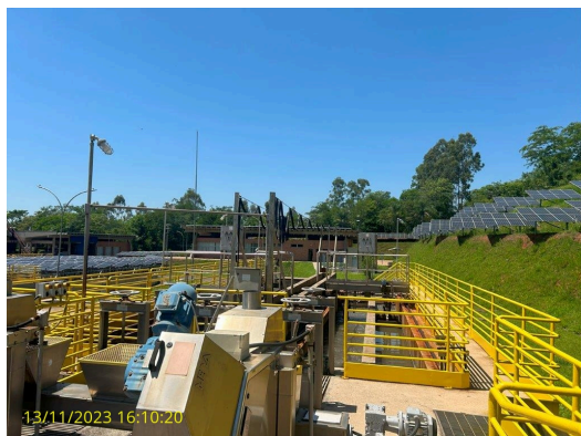
Foto 11 - Gradeamento
