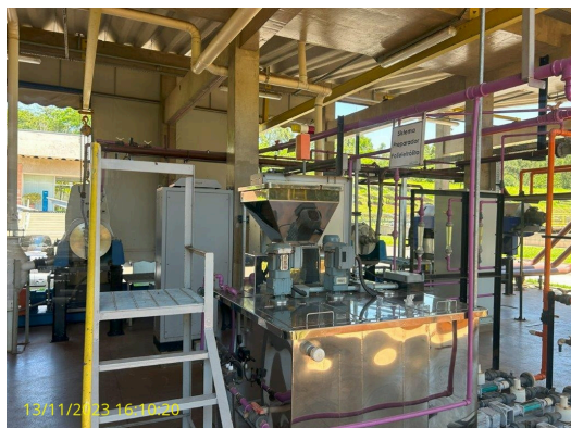
Foto 35 - Preparação de polieletrólito
