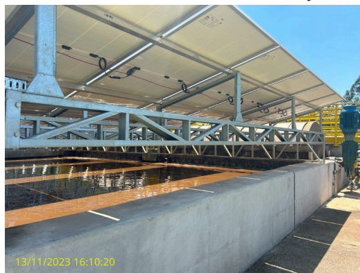
Foto 18 - Placas fotovoltaicas
