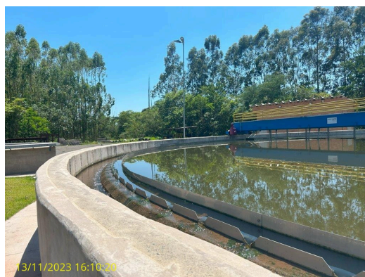
Foto 24 - Decantadores
