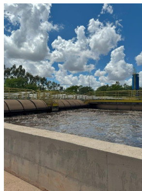
Foto 8 - Reatores aerobios
